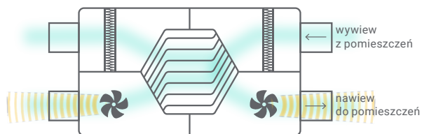
Tradycyjny rekuperator
